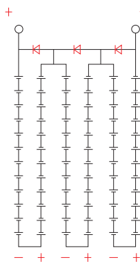
Diagrama de circuito
